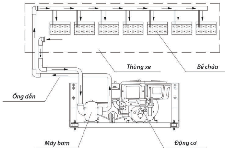
▲ Hình mô tả hệ thống cấp dưỡng khí (máy tạo oxy) để chở thủy sản.
